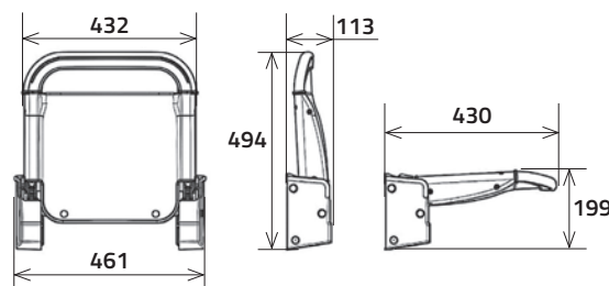
Flip weight 5,7 kg
